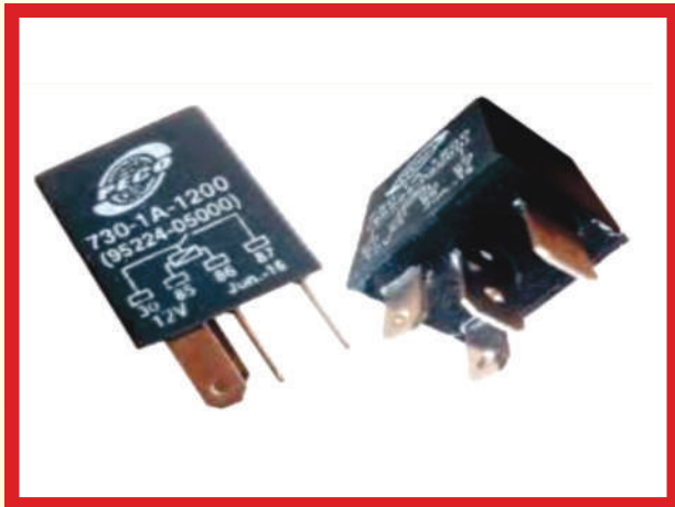
PECO 0138 & PECO 0138/2 Micro Relay 4 Pin 12 V & 24v
